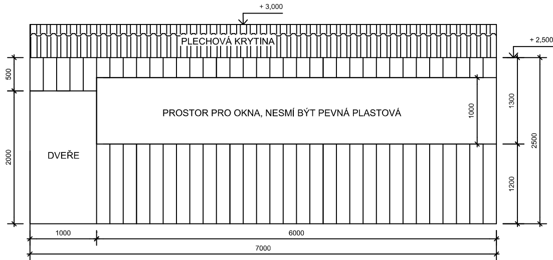
ČELNÍ POHLED - DVEŘE LZE PŘÍPADNĚ ÚMÍSTIT NA DRUHOU STRANU
