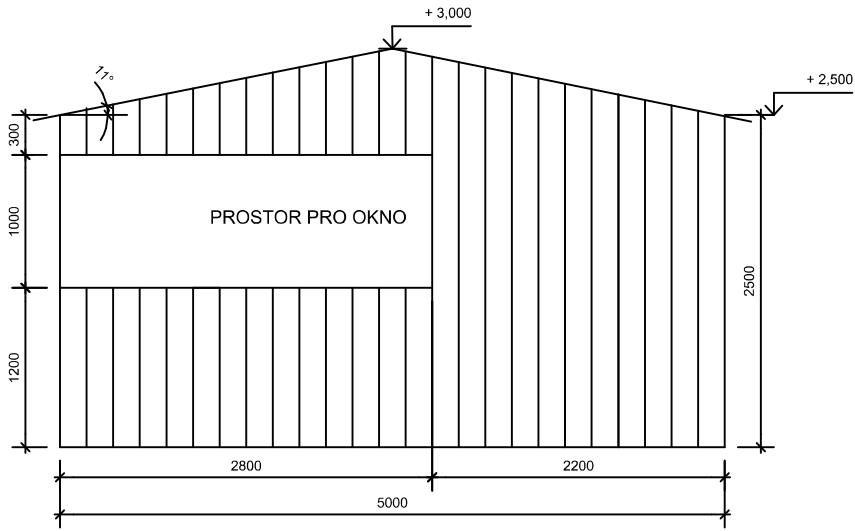
BOČNÍ PRAVÝ POHLED - OKNO NESMÍ BÝT PEVNÉ PLASTOVÉ, PŘÍPADNĚ LZE OKNO ZRUŠIT A MÍT CELOU STRANU PLNĚ OBYTOU, PŘESAŘ STŘECHY MAX DO 200 mm
