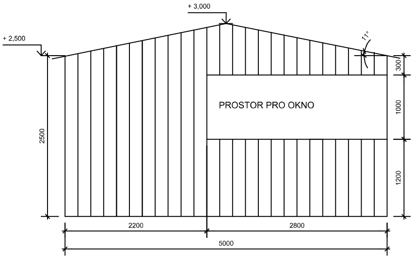
BOČNÍ LEVÝ POHLED - OKNO NESMÍ BÝT PEVNÉ PLASTOVÉ, PŘÍPADNĚ LZE OKNO ZRUŠIT A MÍT CELOU STRANU PLNĚ OBYTOU, PŘESAŘ STŘECHY MAX DO 200 mm
